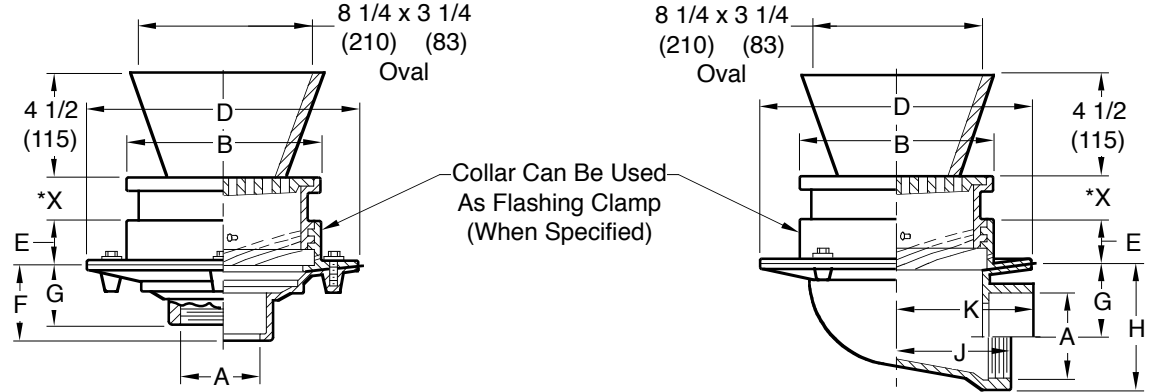
8 1/2"(215) 12"(305) . . . TOP SIZE = B DIA . . . . . 8 1/2"(215) 12"(305) Fig. . . . 3650C . . . 3655C . . . CAULK OUTLET . . . . Fig. . . . 3660C . . . 3665C Fig. . . . 3650T . . . 3655T . . . THREADED OUTLET . . . Fig. . . . 3660T . . . 3665T
